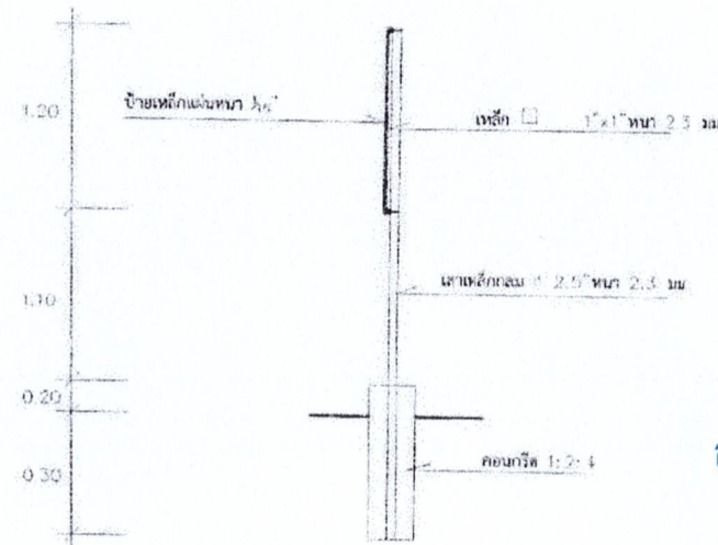
รูปด้านหน้าบ้านประชาชนสัมพันธ์โครงการ
