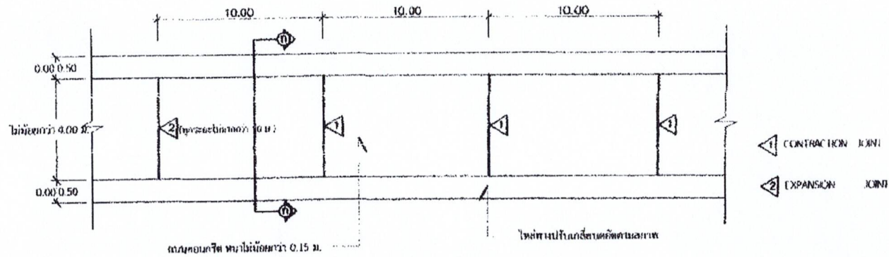
แปลนโครงแบบคอนกรีตเสริมเหล็ก SCALE 1:100
