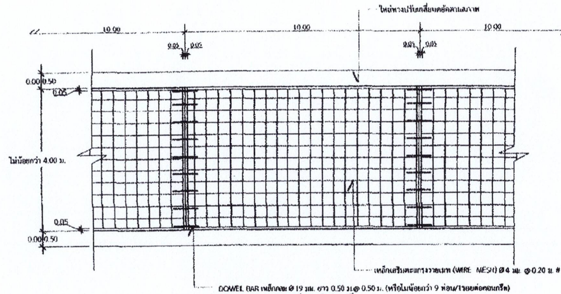
รูปแปลนผิวจากรางคอนกรีตเสริมเหล็ก SCALE 1:50
