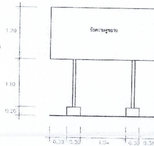
รูปด้านหน้าบ้านประชาชนสัมพันธ์โครงการ
